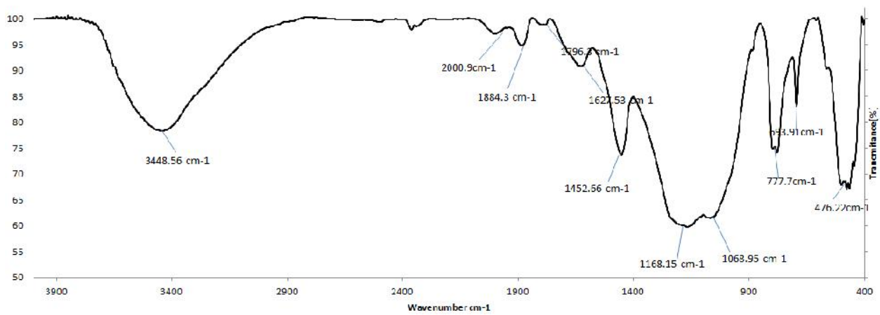
شکل ۵. الگوی FTIR ژئولیت سنتز شده از کاتولین ایرانی
