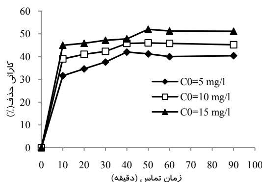
شکل ۲. تأثیر زمان تماس بر روی کارایی حذف Cr(VI) (غلظت اولیه pH=5 ، دوز جاذب ۰.۱g/L، ۰.۵، ۱.۰، ۱.۵ mg/L)
