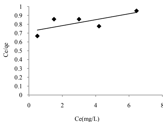
شکل ۷. نمودار \frac{C_e}{q_e} به صورت تابعی از C_e و معادله مشتق از آن بر اساس معادله لانگمویر
