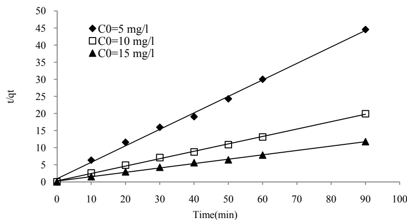
شکل ۶. منحنی سینتیک جذب بر اساس مدل شبه درجه دوم برای جذب کروم
