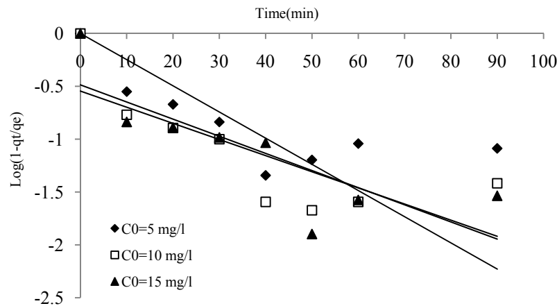
شکل ۵. منحنی سینتیک جذب بر اساس مدل شبه درجه اول برای جذب کروم
