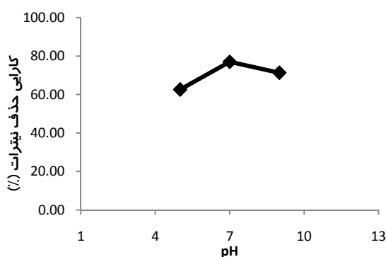
شکل ۳. تأثیر pH بر روی کارایی حذف نیترات (ZnO=۰/۱ g/L, \text{min}
