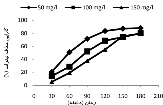
شکل ۱. تأثیر زمان تماس در غلظت‌های اولیه نیترات بر حسب میلی گرم در لیتر (ZnO=۰/۱ g/L, \text{pH}=7 )
