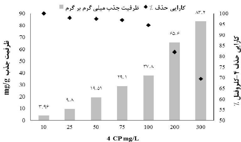
نمودار ۴. تاثیر تغییرات غلظت ۴-کلروفنل (pH اولیه محلول: ۱۱، pH شرایط اصلاح: ۵/۴، دوز جاذب ۲/۲۵ g، میزان اصلاح ۲ برابر CEC، زمان تعادل: ۱۲۰ min)
