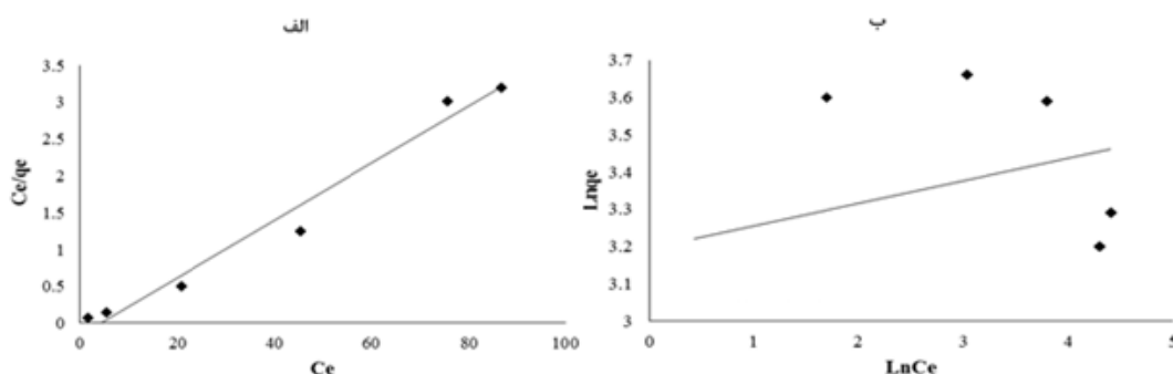
نمودار ۵. ایزوترم‌های جذب قسمت الف و ب، به ترتیب ایزوترم جذب لانگمیر و فروندلیچ (pH اولیه محلول: ۱۱، pH شرایط اصلاح: ۴/۵، میزان اصلاح ۲ برابر CEC، ۴-کلروفنل ۱۰۰ mg/L، زمان تعادل: ۱۲۰ min)
