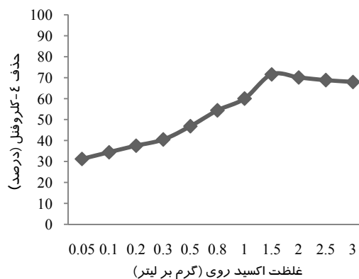
شکل ۳. تاثیر دوز اکسید روی بر کارایی حذف E-کلروفنل (pH=9) غلظت اولیه E-کلروفنل=۱۰۰ میلی گرم در لیتر
