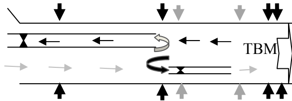
شکل ۳. تهویه کمکی با اورلاپ ضعیف
