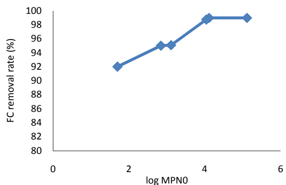
نمودار ۲. تأثیر دز اولیه باکتری در راندمان گندزدایی به وسیله \text{Fe}_3\text{O}_4@\text{C}@\text{Ag} غلظت گندزدا ۶۰ mg/L برحسب نقره، زمان تماس ۳۰ دقیقه
