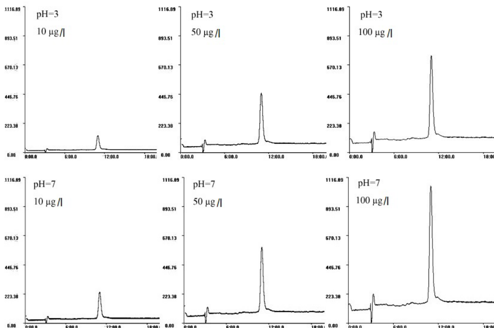
شکل ۳. نمایش اختلاف سیگنال‌های بازیابی ونکومایسین از محیط آبی در غلظت‌های ۱۰، ۵۰ و ۱۰۰ میکروگرم در لیتر در pH‌های ۳ و ۷
