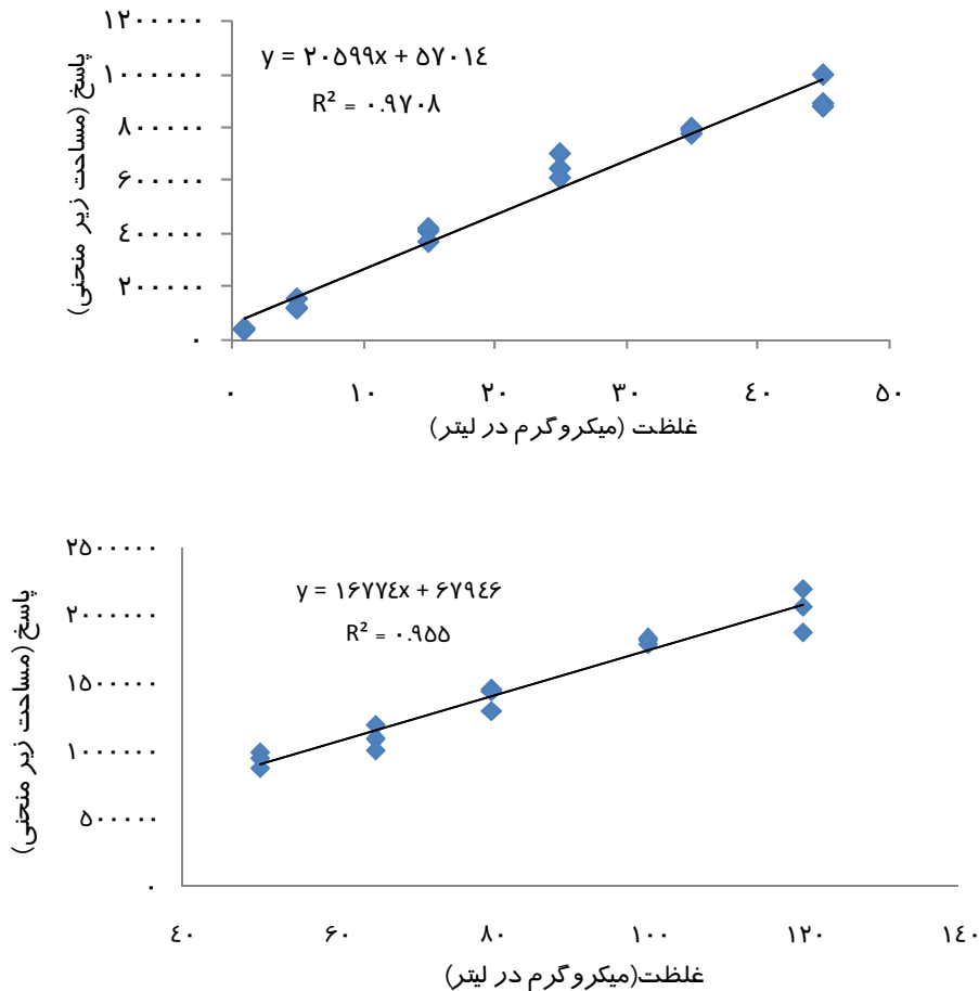
شکل ۵. منحنی‌های کالیبراسیون رسم شده برای آنالیز نکومایسین در محدوده غلظت‌های ۱ الی ۴۵ و ۵۰ الی ۱۲۰ میکروگرم در لیتر
