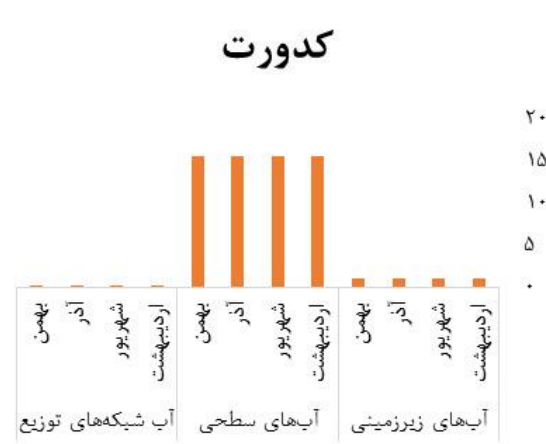
شکل ۵. میانگین غلظت کدورت (NTU) در منابع آب استان اردبیل بر حسب فصول سال
