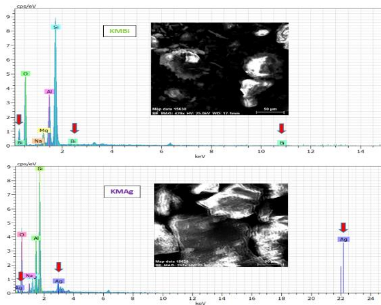
شکل ۴. نتیجه آنالیز SEM/EDX نمونه‌های نانورس تیمار شده با یون‌های نقره (KMAg) و بیسموت (KMBi)
