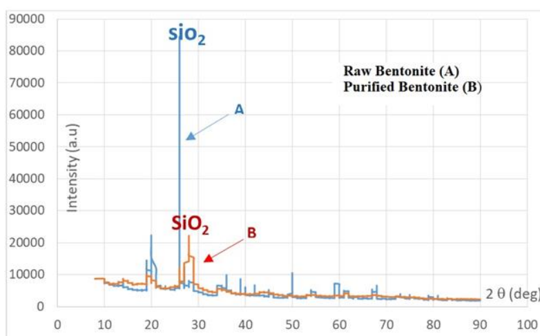
شکل ۲. الگوهای پراش اشعه ایکس بنتونیت خام (A) و بنتونیت خالص شده (B)
