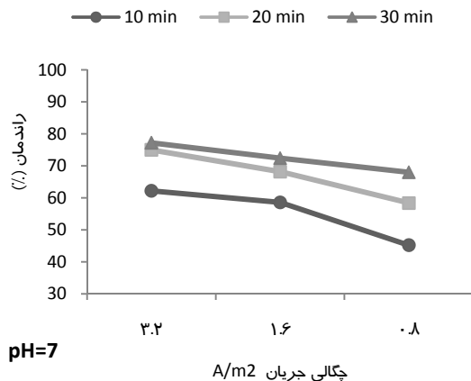
نمودار ۲. راندمان حذف کدورت بوسیله انعقاد الکتریکی با الکترودهای آهن در pH خنثی
