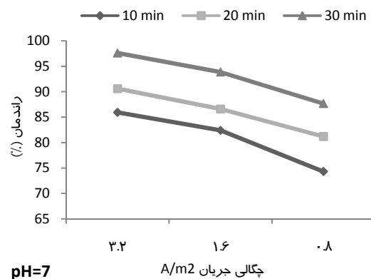
نمودار ۱. راندمان حذف کدورت بوسیله انعقاد الکتریکی با الکترودهای آلومینیوم در pH خنثی
