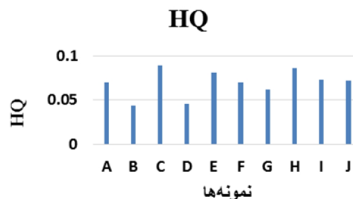
شکل ۵. خطر غیر سرطان‌زایی فرمالدئید در هوای داخلی سالن‌های زیبایی زنانه شهر گناباد
