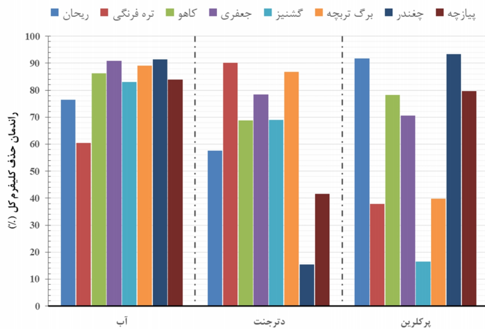
مراحل گندزدایی سبزیجات نمودار ۱. میزان راندمان حذف کلیفرم کل توسط مراحل مختلف گندزدایی در نمونه‌های سبزیجات
