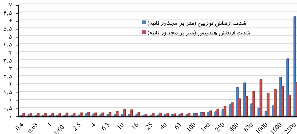
شکل ۶. تجزیه فرکانسی یک سوم اکتاوباند (هرتز) شتاب ارتعاش ابزارهای دندانی‌شکی (هندپیس و توربین)
