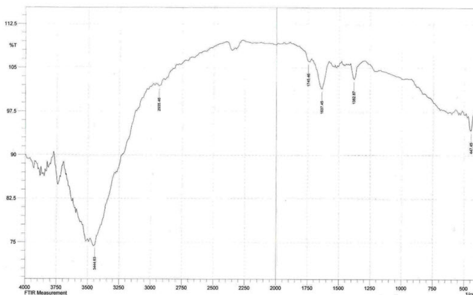
شکل ۳. تصویر FTIR نانوذرات نقره سنتز شده به روش انفجار الکتریکی سیم
