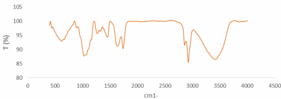
شکل ۲. تصویر FTIR از جاذب تهیه شده از پودر آلوتیورای اصلاح شده با اسید سولفوریک
