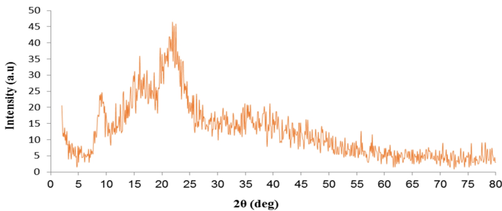
شکل ۳. تصویر XRD از جاذب تهیه شده از پودر آلوتیورای اصلاح شده با اسید سولفوریک
