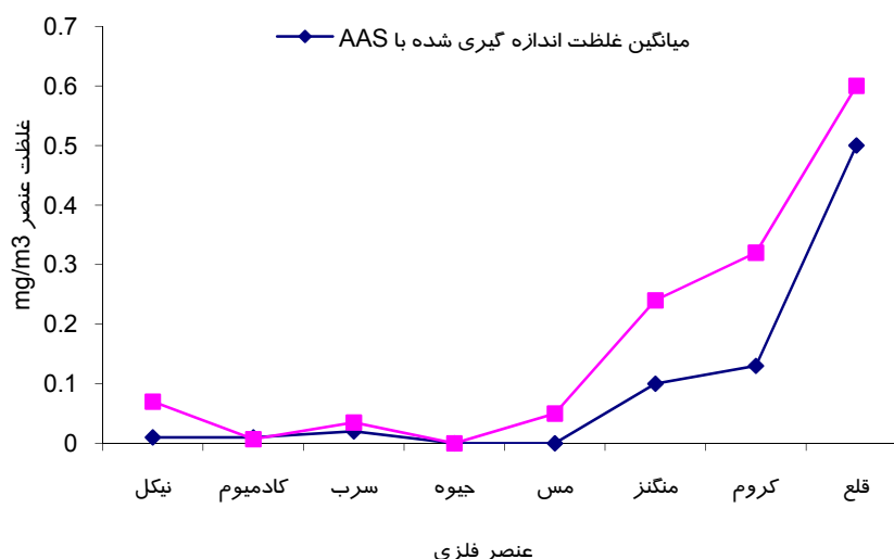
نمودار ۱. مقایسه میانگین غلظت فیوم های ناشی از برش فلزات قراضه با استفاده از دو روش طیف سنجی جذب اتمی (AAS) و طیف سنجی نشر اتمی با پلاسمای کوپل شده القائی (ICP-AES)
