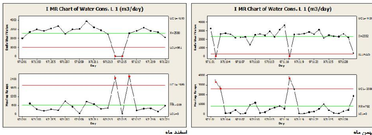
شکل ۱. نمودارهای کنترلی مصرف آب خط ۱ در سال ۱۳۹۷: نمودار کنترل فرایند (پایین) و نمودار کنترل نمونه (بالا)
