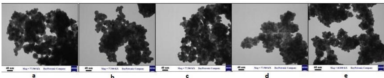
شکل ۵. تصاویر TEM مربوط به نانوذرات سنتز شده به روش سل-ژل: (a) ZnO (b) Mg5%-La5%/ZnO (c) La4%/ZnO (d) Mg5%-La5%/ZnO (e) Mg6%-La4%/ZnO
