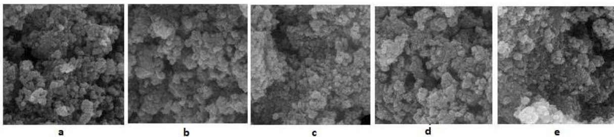
شکل ۴. تصاویر FESEM مربوط به نانوذرات سنتز شده به روش سل-ژل: (a) ZnO (b) Mg5%-La5%/ZnO (c) La4%/ZnO (d) Mg5%-La5%/ZnO (e) Mg6%-La4%/ZnO
