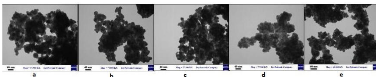
شکل ۵. تصاویر TEM مربوط به نانوذرات سنتز شده به روش سل-ژل: Mg6%-La4%/ZnO (e) و Mg5%-La4%/ZnO (d)، La4%/ZnO (c)، Mg5%/ZnO (b)، ZnO (a)
