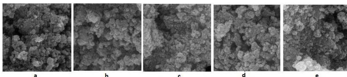
شکل ۴. تصاویر FESEM مربوط به نانوذرات سنتز شده به روش سل-ژل: Mg6%-La4%/ZnO (e) و Mg5%-La4%/ZnO (d)، La4%/ZnO (c)، Mg5%/ZnO (b)، ZnO (a)
