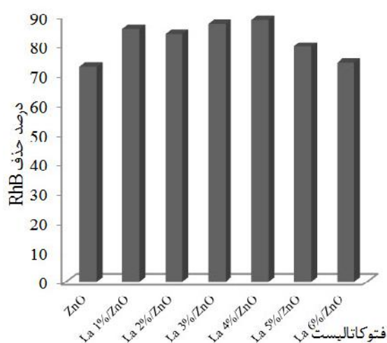
نمودار ۲. مقایسه درصد حذف RhB با نانوذرات \text{ZnO} و \text{LaX\%/ZnO} ( X=1-6\% ) ۲۱ دقیقه تابش اشعه UVC
