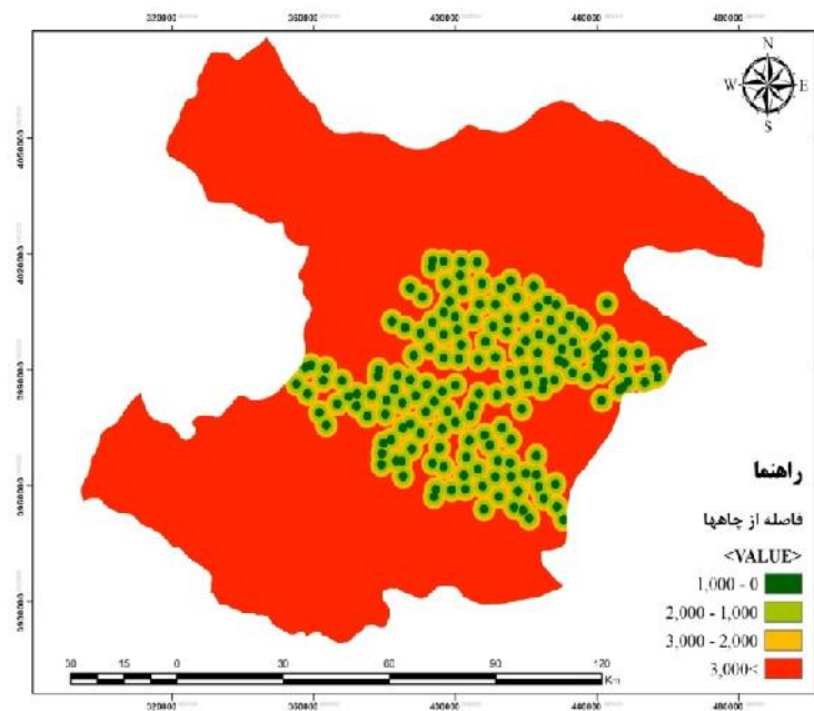
شکل ۱۰. نقشه فاصله از چاه‌های آب‌های زیرزمینی
