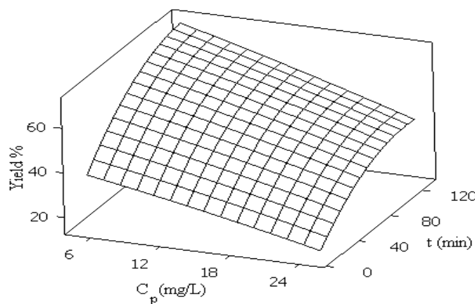
شکل ۳. پاسخ سطحی % راندمان در برابر دما و زمان (مقدار جاذب: ۳/۷۸ گرم، دما: ۲۰ °C، pH=۳/۶۳)
