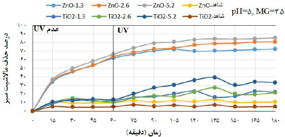
شکل ۵. درصد حذف مالاشیت سبز در غلظت ۳/۵ میلی‌گرم بر لیتر و pH=۵
