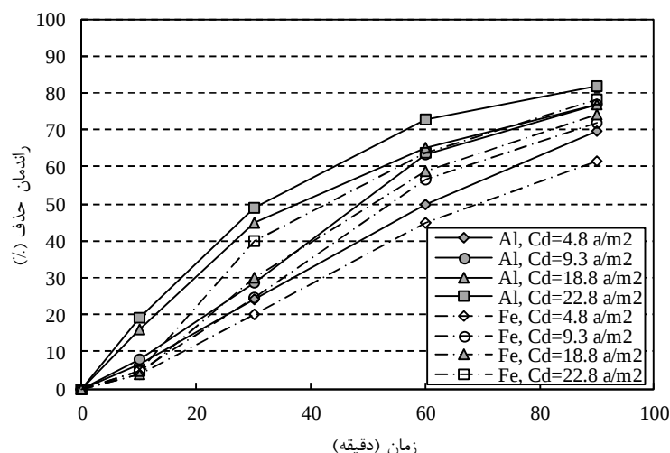
شکل ۲. اثر دانسیته جریان بر روی حذف نیترا ت (غلظت اولیه نیترا ت 125 \text{ mg/l} ، \omega = 1.8 \text{ rpm} )
