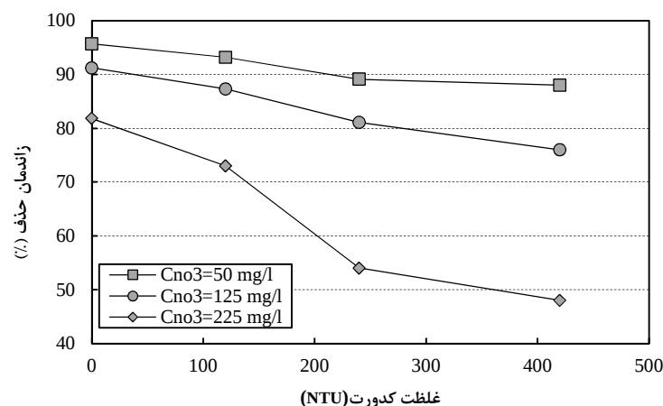
شکل ۶. تاثیر مقادیر متفاوت کدورت بر روی راندمان حذف نیترات (الکتروآلومینیومی، دانسیته جریان 22/8 \text{ A/m}^2 ، سرعت چرخش 8/2 \text{ rpm} و زمان ۹۰ دقیقه)
