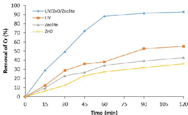
نمودار ۴. تاثیر ZnO، زئولیت، UV و UV/ZnO-Zeolite به تنهایی در حذف فتوکاتالیستی کروم شش ظرفیتی: 30 \text{ mg/l} ( \text{pH}=5 ، مقدار کامپوزیت 1/5 \text{ g/L} ، غلظت اولیه کروم شش ظرفیتی: 30 \text{ mg/l} )
