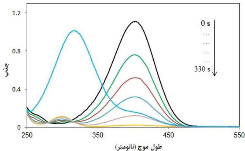
شکل ۷. طیف UV-Vis از محلول آبی ۴- نیتروفنول در حضور ۲۵۰ میلی مولار \text{NaBH}_4 و ۱۰/۰ میلی گرم نانو کامپوزیت نقره- اکسید روی بیوستنزشده (منحنی های رنگی در طول موج ۴۰۰ نانومتر، کاهش پیک جذبی مربوط به ۴- نیتروفنول را در طی واکنش حذف نشان می دهند).
