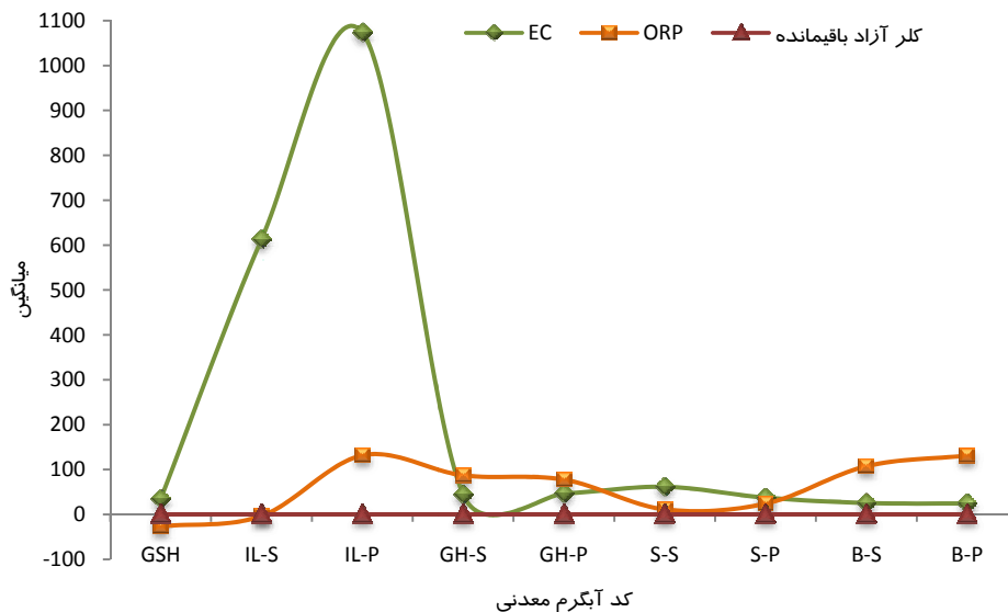
نمودار ۲. میانگین هدایت الکتریکی آب (EC (μMho/cm)، کلر آزاد باقیمانده (mg/L) و پتانسیل ردوکس (ORP (mV)) در آبگرمهای معدنی شهرستان نیر در طول دوره تحقیق
