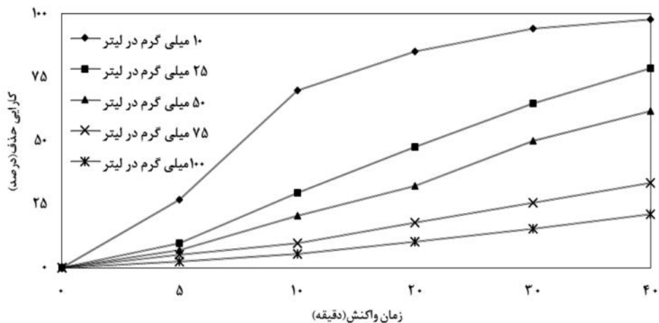
نمودار ۴. تأثیر غلظت اولیه SDBS نسبت به زمان بر کارایی فرایند (pH=3): غلظت آنیون پرسولفات ۵۰ میلی مولار؛ غلظت ازن ۵ میلی گرم در لیتر در نمودار ۴. تأثیر غلظت اولیه SDBS نسبت به زمان بر کارایی فرایند (pH=3): غلظت آنیون پرسولفات ۵۰ میلی مولار؛ غلظت ازن ۵ میلی گرم در لیتر در نمودار ۴.
