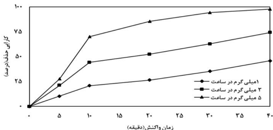
نمودار ۳. تاثیر غلظت ازن ورودی نسبت به زمان بر کارایی فرایند (غلظت اولیه SDBD=۱۰ میلی گرم در لیتر؛ pH=3؛ غلظت آنیون پرسولفات=۵۰ میلی مول بر لیتر)
