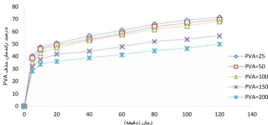
شکل ۷. تعیین تأثیر تغییرات غلظت اولیه پلی‌وینیل الکل در فرایند \text{Mn}_3\text{O}_4/\text{H}_2\text{O}_2 در حذف پلی‌وینیل الکل ( \text{pH} ۳، غلظت کاتالیست 0.4 \text{ g/L} و غلظت \text{H}_2\text{O}_2 برابر با 20 \text{ mmol/L} )
