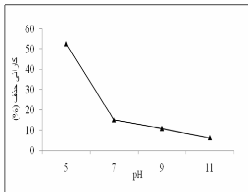
شکل ۴. بررسی تأثیر pH بر روی کارایی حذف رنگ Acid Red 18 (در حضور ۰/۸ گرم کربن فعال در ۲۰۰ سی سی نمونه با غلظت ۱۰۰ mg/L)
