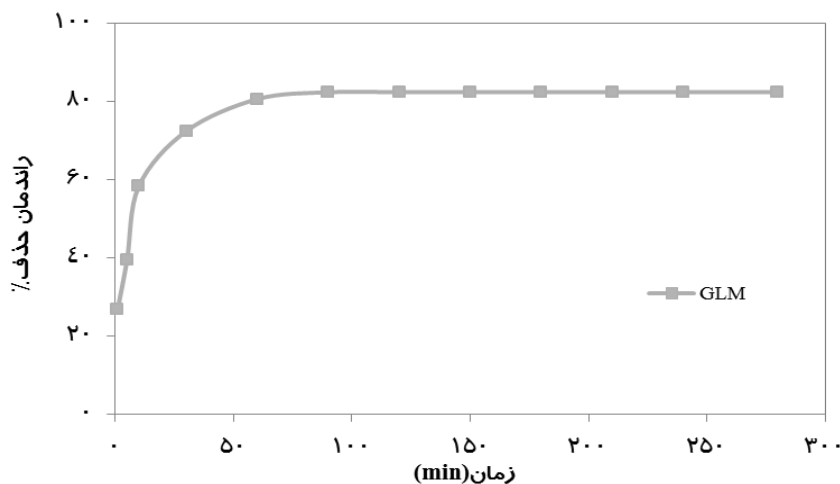
شکل ۴. اثر زمان تماس (غلظت اولیه نیترات ۲۵mg/l، دوز جاذب ۴g/l، pH اولیه محلول ۷ و سرعت ۱۵۰ دور بر دقیقه)
