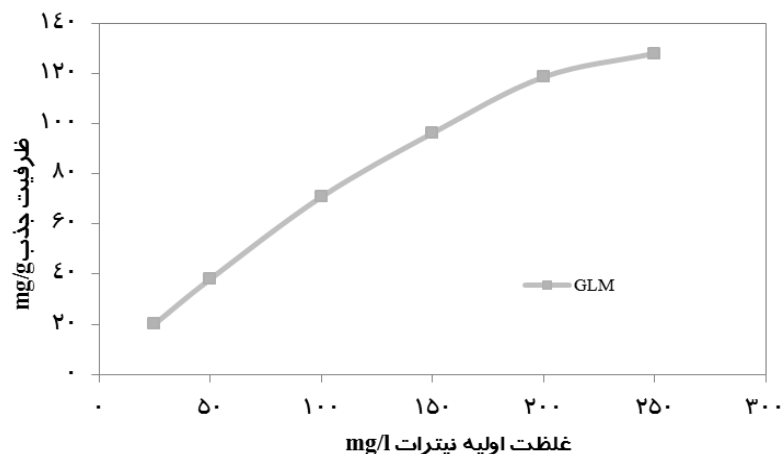
شکل ۳. اثر غلظت اولیه نیترات (دوز جاذب ۴g/l؛ زمان تماس ۶۰ دقیقه، pH اولیه محلول ۷ و سرعت ۱۵۰ دور بر دقیقه)
