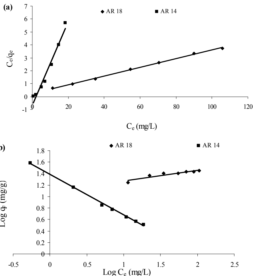
شکل ۵. نتایج حاصل از مطالعه ثابت تعادل، (a) مدل ایزوترمی لانگمویر، (b) مدل ایزوترمی فروندلیخ
