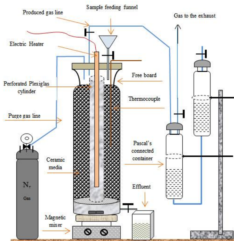
شکل ۱. شماتیک بیورآکتور استفاده شده برای حذف سولفات و ترسیب مس
