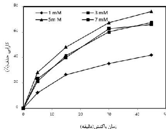
شکل ۴. تاثیر غلظت های مختلف پراکسید هیدروژن بر راندمان الکتروفتون (غلظت اولیه ۴ کلروفنل ۵۰، ۳ mg/L، pH=۵، دانسیته جریان ۳ mA/cm 2 ، زمان ۴۵ min)
