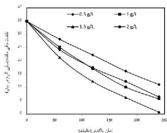
شکل ۷. تاثیر دز مختلف دی اکسید تیتانیوم بر راندمان فتوکاتالیستی (غلظت اولیه ۴ کلروفل ۳۵mg/L، pH=۵/۸، زمان ۲۴۰ min)
