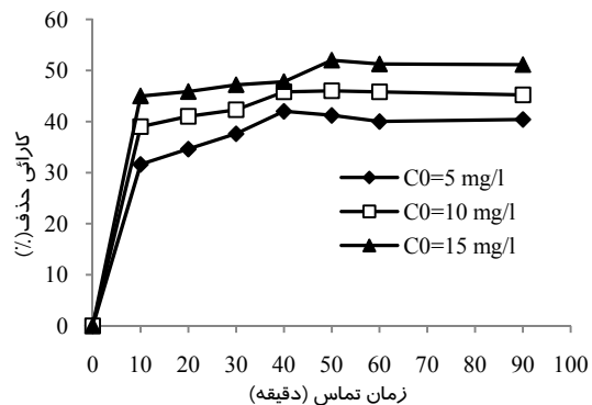
شکل ۲. تأثیر زمان تماس بر روی کارایی حذف Cr(VI) (غلظت اولیه ۵، ۱۰، ۱۵ mg/L دوز جاذب ۰.۱g/L، pH=۵)
