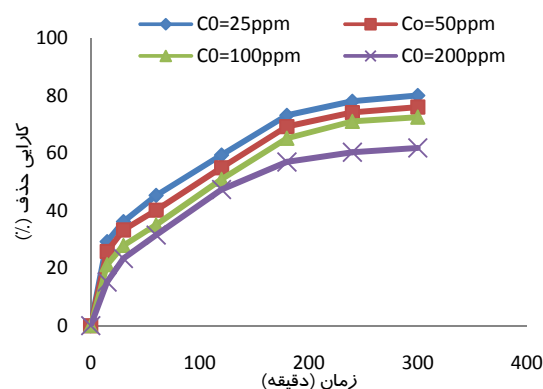
شکل ۵. مقایسه راندمان حذف در غلظت‌های مختلف E-کلروفنل (۲۵، ۵۰، ۱۰۰، ۲۰۰ میلی گرم در لیتر توسط فرایند فتوکاتالیستی (pH=9)، دوز اکسید روی: ۱/۵ گرم در لیتر)
