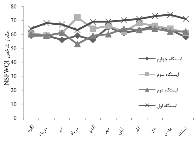
شکل ۸. نمودار تغییرات زمانی میزان NSFQI در طول رودخانه هیرو چایی در دوره نمونه برداری در ایستگاه‌های مختلف
