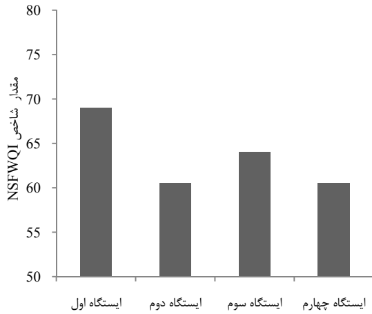
شکل ۹. نمودار تغییرات مکانی میانگین شاخص NSFQI در طول رودخانه هیرو چایی در دوره نمونه برداری در ایستگاه‌های مختلف
