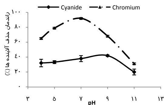
شکل ۱. راندمان حذف همزمان آلاینده‌های سیانید و کروم بر حسب میزان pH (غلظت‌های اولیه کروم و سیانید برابر با ۱۰ mg/L و FeCl 3 =۰.۷g/L و زمان ته نشینی ۶۰ دقیقه)
