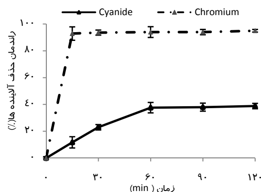
شکل ۳. تاثیر زمان بر راندمان حذف همزمان آلاینده‌های سیانید و کروم (غلظت‌های اولیه کروم و سیانید برابر با 10 \text{ mg/L} ، pH=7 و \text{FeCl}_3=0.7 \text{ g/L} )
