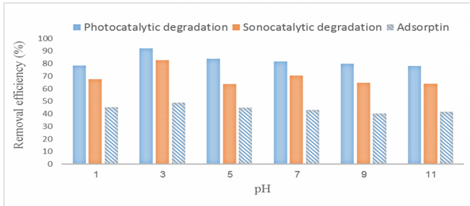
شکل ۷. تأثیر pH بر میزان کارایی حذف ۲-کلروفنول در حضور نانوذرات اکسیدروی سنتز شده از گل کاغذی طی فرایندهای فتوکاتالیستی و سونوکاتالیستی و مقایسه آن‌ها با فرایند حذف توسط جذب سطحی در یک شرایط تاریک
