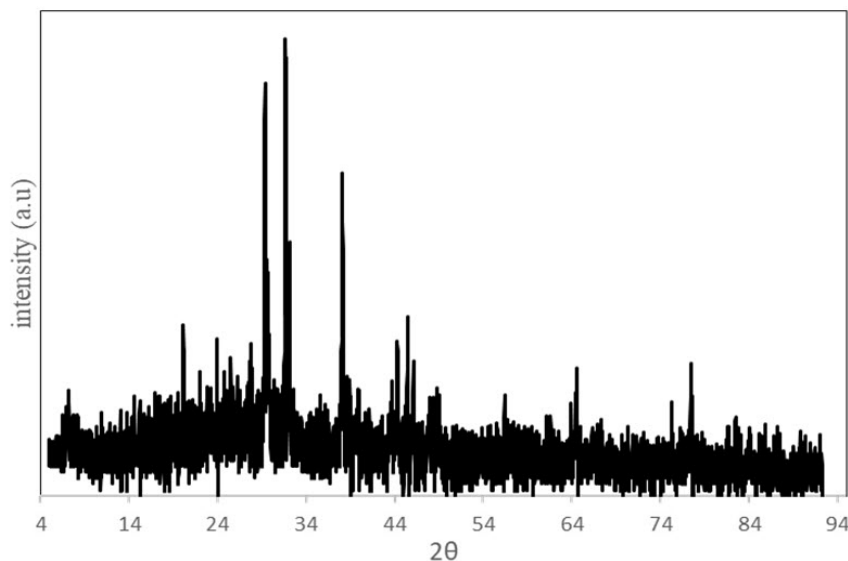
شکل ۲. تصویر XRD نانوذرات نقره سنتز شده به روش انفجار الکتريکی سیم
