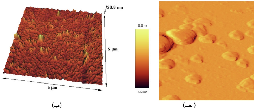
شکل ۴. تصاویر AFM از نانوذرات نقره سنتز شده به روش انفجار الکتریکی سیم (الف) تصویر سه بعدی (ب) تصویر دو بعدی
