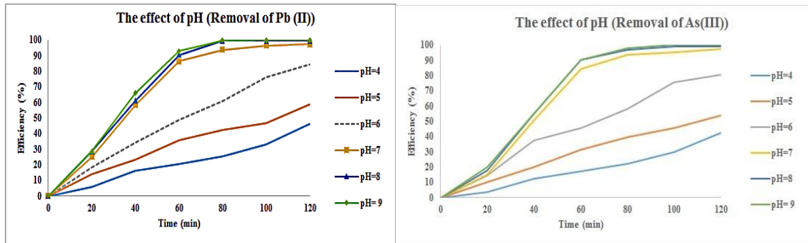
شکل ۶. تأثیر مقدار pH بر کارایی نانوفتوکاتالیزوری در غلظت اولیه آلاینده برابر با ۵ mg.L -1
