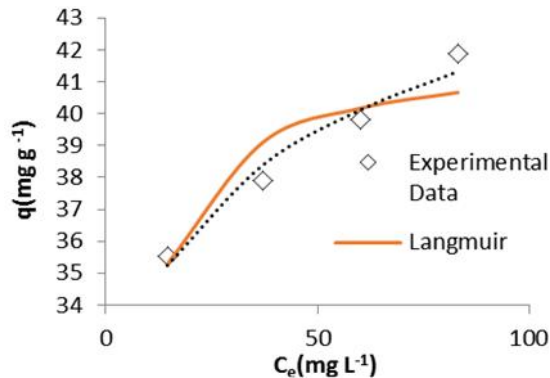
شکل ۶. مقایسه نتایج نمودار مدل ایزوترم جذب سطحی لانگموئیر و فروندلیچ با داده‌های تجربی در pH=4 برای حذف آرسنیک
