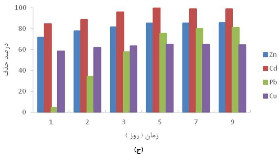
نمودار ۲. حذف فلزات سنگین از لجن فاضلاب شهری با استفاده از شستشوی بیولوژیکی در مقادیر مختلف آهن (الف=۱ Fe gr/l)، (ب=۲ Fe gr/l) و (ج=۴ Fe gr/l)
