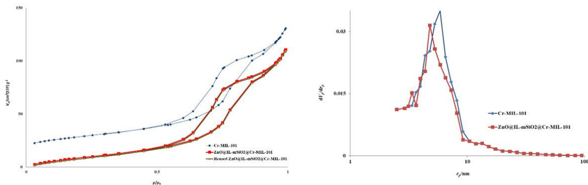
شکل ۳. ایزوترم جذب/ دفع نیتروژن و تجزیه و تحلیل BJH مربوط به، Cr-MIL-101 و نانوفتوکاتالیزور ZISM
