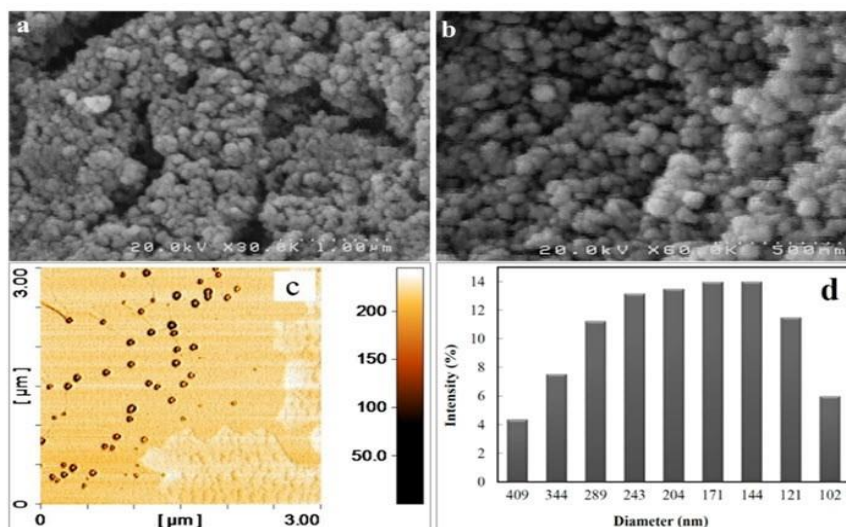
شکل ۲. SEM (a و b) و AFM (c) و DLS (d) مربوط به نانوفتوکاتالیزور ZISM
