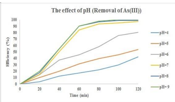
شکل ۶. تأثیر مقدار pH بر کارایی نانوفتوکاتالیزوری در غلظت اولیه آلاینده برابر با 5 \text{ mg.L}^{-1}
