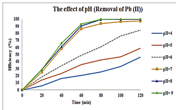
شکل ۶. تأثیر مقدار pH بر کارایی نانوفتوکاتالیزوری در غلظت اولیه آلاینده برابر با 5 \text{ mg.L}^{-1}
