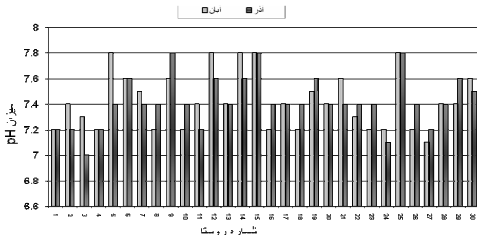
نمودار ۲. میزان pH در شبکه آبرسانی روستاهای مورد بررسی اردبیل در ماههای آبان و آذر در سال ۱۳۸۹
