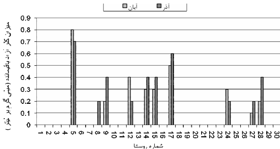
نمودار ۱. میزان کلر باقیمانده در شبکه آبرسانی روستاهای مورد بررسی اردبیل در ماههای آبان و آذر در سال ۱۳۸۹
